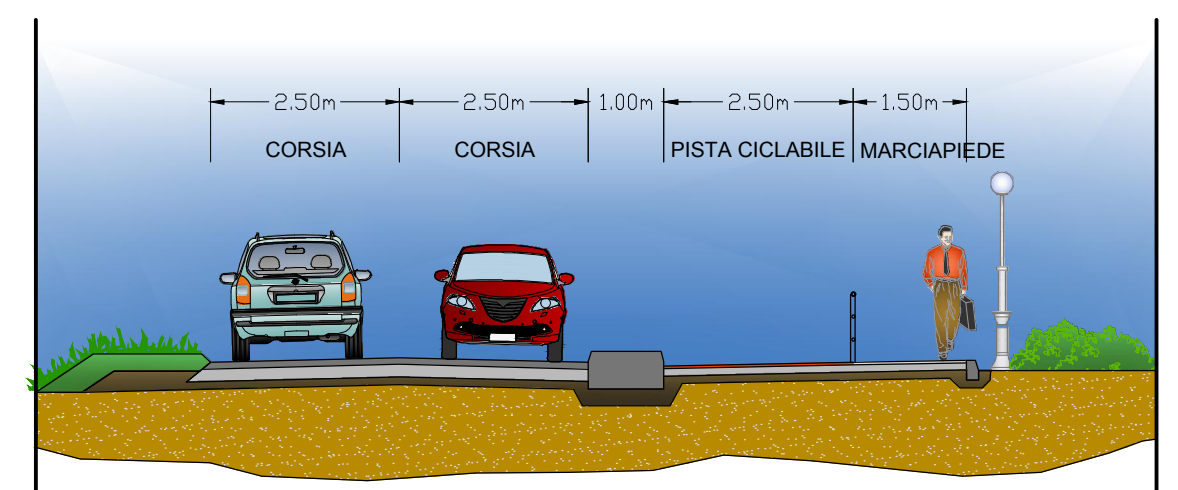
PERCORSO CICLOPEDONALE AFFIANCATO ALLA VIABILITA'
