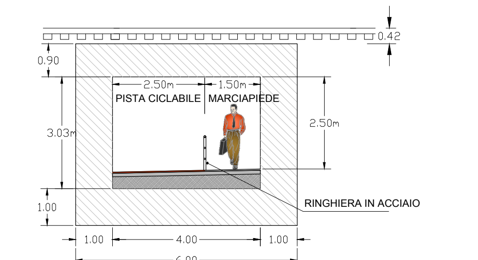
PERCORSO CICLOPEDONALE AFFIANCATO ALLA VIABILITA'
