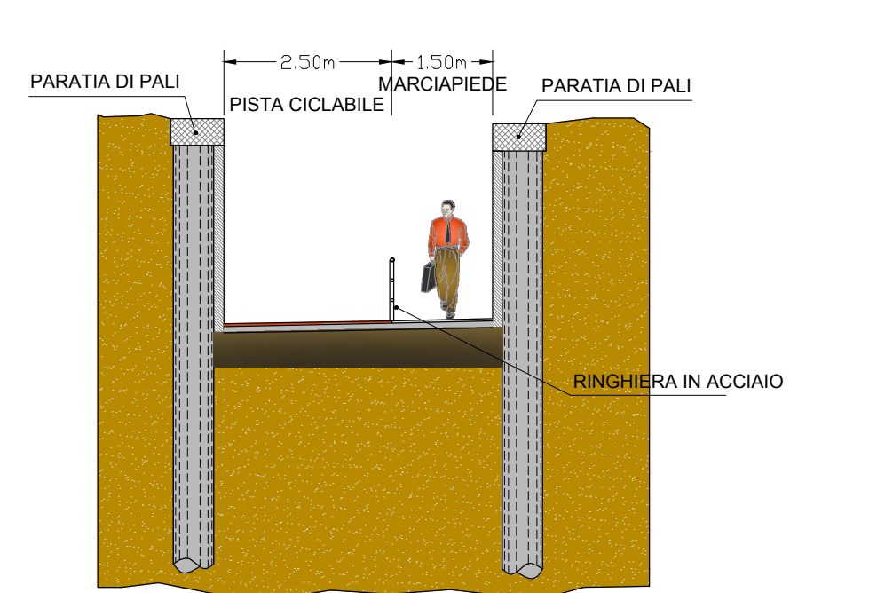
PERCORSO CICLOPEDONALE TRA PARATIE
